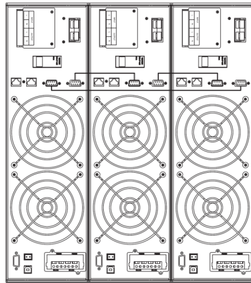
Παράλληλο σύστημα με 3 UPS
