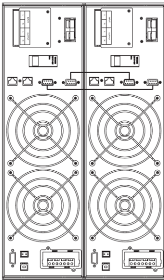
Παράλληλο σύστημα με 2 UPS
